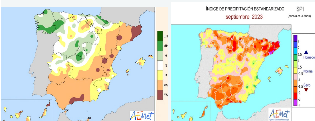
GRÁFICO 1 Precipitaciones en 2023
